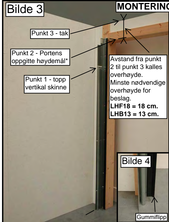
Bilde 3. Høydetilpasning og eventuell kapping eller heving av karmvinkel og vertikal løpeskinne. Avstanden fra gulvet til toppen av vertikale løpeskinne (punkt 1) skal være portens oppgitte høyde -33 cm. Er overhøyde større en 18 cm for type LHF18 eller 13 cm for type LHB13, kan målet -33 cm reduseres tilsvarende inntil -29 cm eller skinnen kan heves inntil 3 cm fra gulvet. Porten kommer dermed nærmere taket i åpen stilling. Kapp skinnen og karmvinkel i bunn om nødvendig. Kontroller følgende før karmvinkelen skrues fast. Avstanden fra punkt 1 til punkt 3 for type LHF18 må min. være 51 cm, for type LHB13 min. 46 cm. Portens oppgitte høydemål se vedlagt gjenkjenningssmerke.
