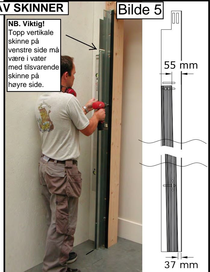
Bilde 4. Før karmvinkel med løpeskinne festes til veggen må tettelist monteres til karmvinkelen. Gummi flippet skal vende innover for å gi best tetting mot porten. Bilde 5. Plasser den ferdig tilpassede skinnen med karmvinkelen på streken. Skru fast nederst med 1 stk. 40 mm fransk treskrue. Bruk vater for å sette karmvinkelen i lodd og skru fast i topp og på midten. NB. Viktig! toppen av vertikal skinne på den ene siden må være i vater med toppen av skinnen på den andre siden. Juster vertikal løpeskinne så avstanden nederst mellom vertikal løpeskinne og karmvinkel ut/inn er lik ca.35 mm. Skinnen skal i toppen helle innover i garasjen. Avstanden i toppen av vertikale skinnen og karmvinkel skal være 55 mm. Skal senere finjusteres.
