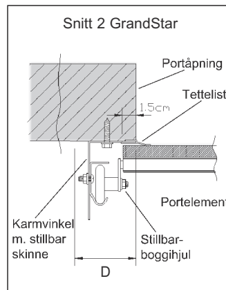
Snitt av port og sidekarmer sett ovenfra som viser tetning og nødvendig sideklaring.
